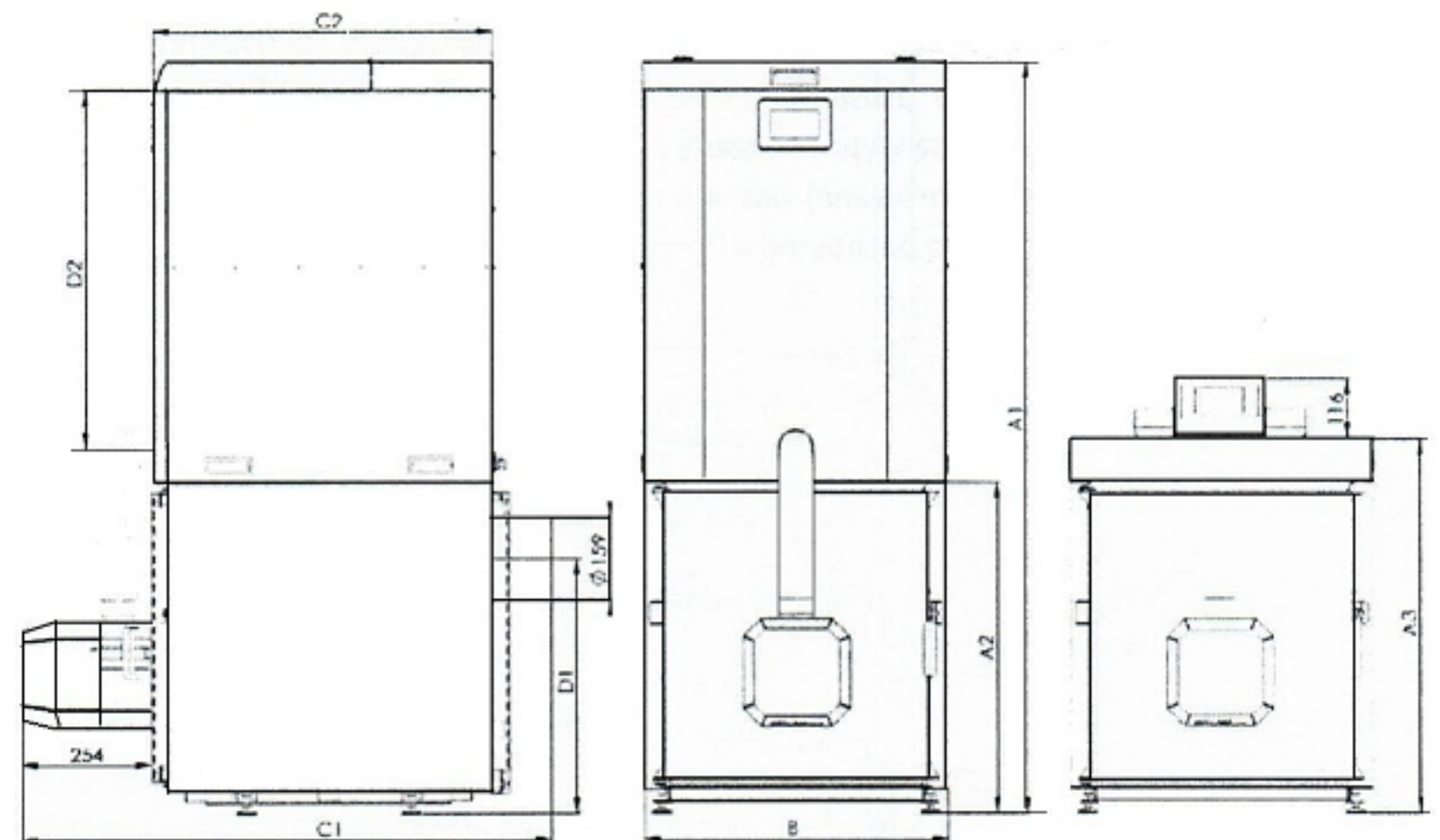
Zestawienie wymiarów gabarytowych
