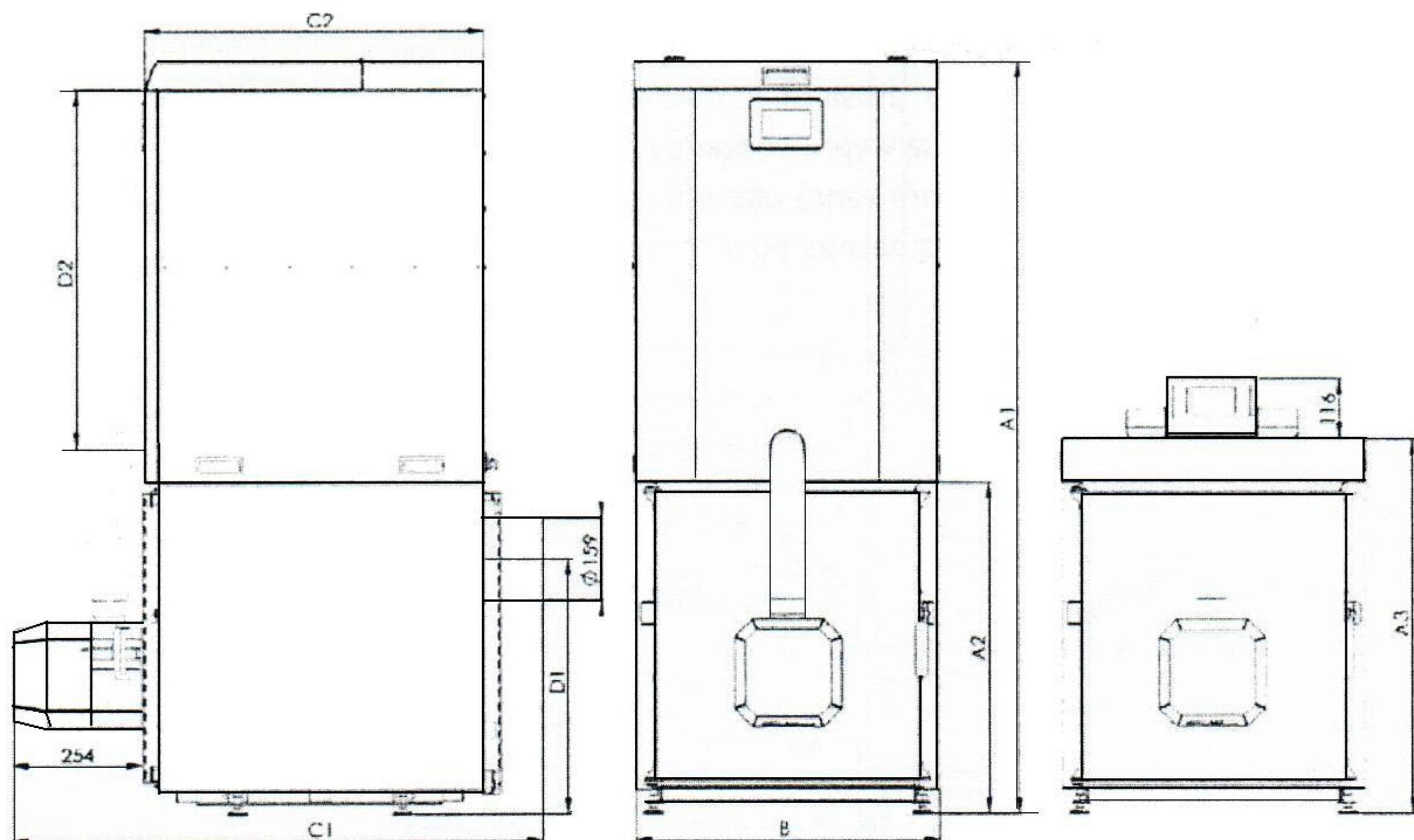
Rysunek 8 – Wymiary gabarytowe kotła
